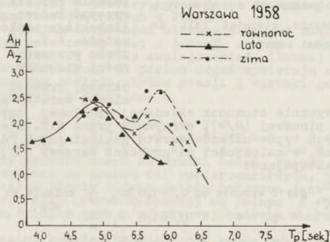
Fig. 2. Krzywe zależności stosunku amplitud poziomych do pionowych ( A_H/A_Z ) od okresu ( \tau ) dla drgań mikrosejsmicznych rejestrowanych przez stację Warszawa
