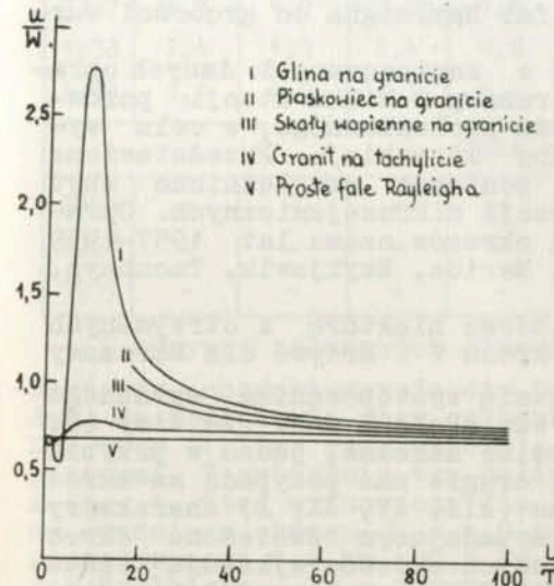
Fig. 1. Krzywe zależności stosunku przesunięć poziomych do pionowych \frac{u}{w} od stosunku długości fali do grubości warstwy \frac{L}{T}
