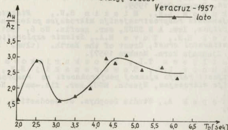
Fig. 5. Krzywa zależności stosunku amplitud poziomych do pionowych ( A_H/A_z ) od okresu ( \tau ) dla drgań mikrosejsmicznych rejestrowanych przez stację Veracruz
