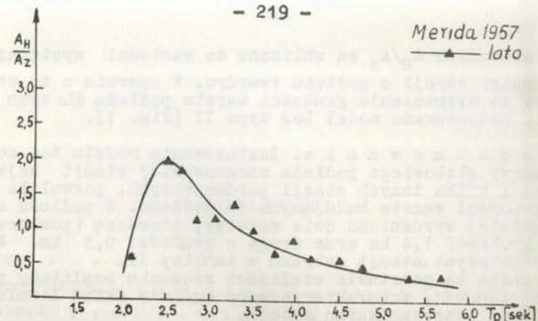
Fig. 3. Krzywa zależności stosunku amplitud poziomych do pionowych ( A_H/A_z ) od okresu ( \tau ) dla drgań mikrosejsmicznych rejestrowanych przez stację Merida
