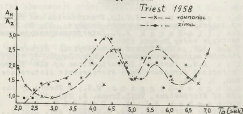
Fig. 4. Krzywe zależności stosunku amplitud poziomych do pionowych ( A_H/A_z ) od okresu ( \tau ) dla drgań mikrosejsmicznych rejestrowanych przez stację Trieste
